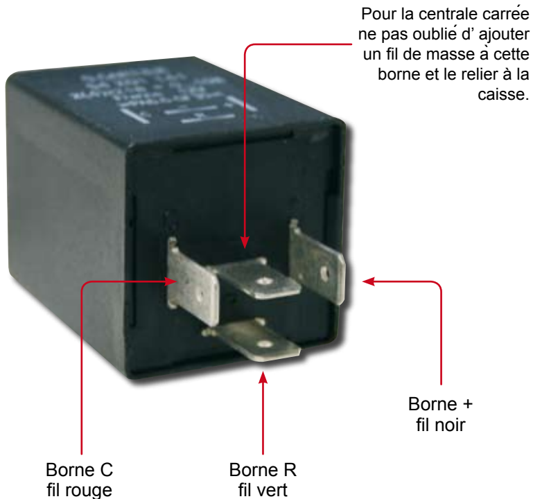
Centrale clignotante carrée
